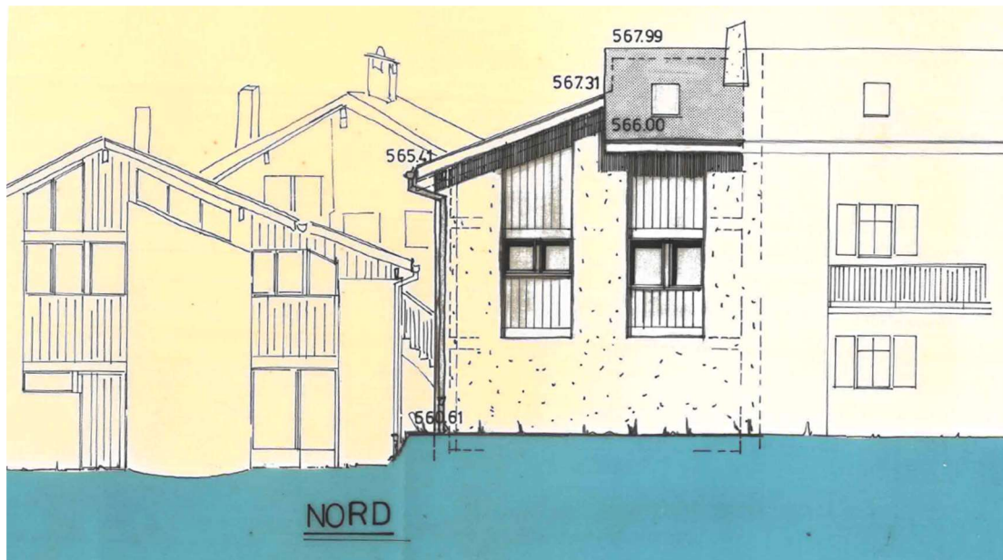
Plans de la maison - coupe
